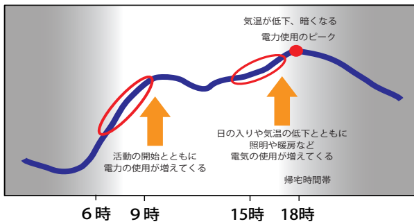
冬の一般的な電力の使用状況
