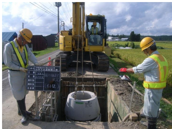
マンホール立込状況
