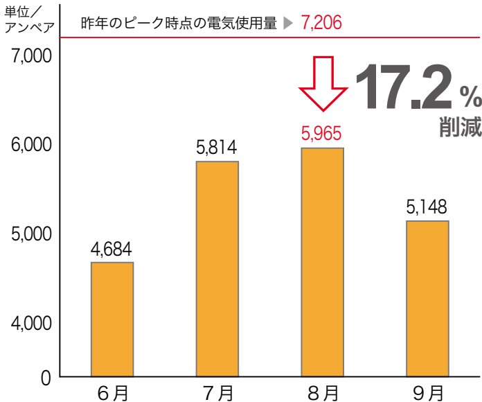
グラフ/取り組み期間各月のピーク時点の電気使用量
