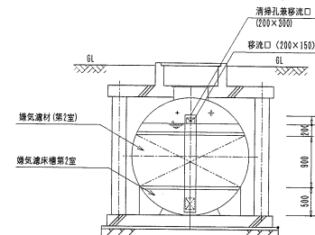
C-C 断面図
