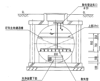
D-D 断面図
