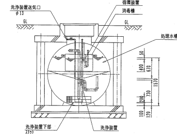
E-E 断面図
