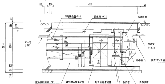
A-A 断面図
