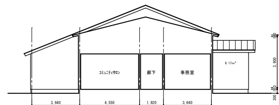
E-E 断面図 S=1/100
