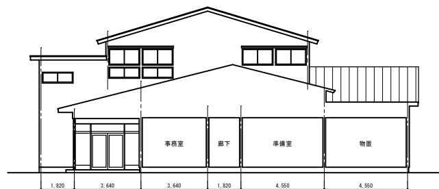
C-C 断面図 S=1/100
