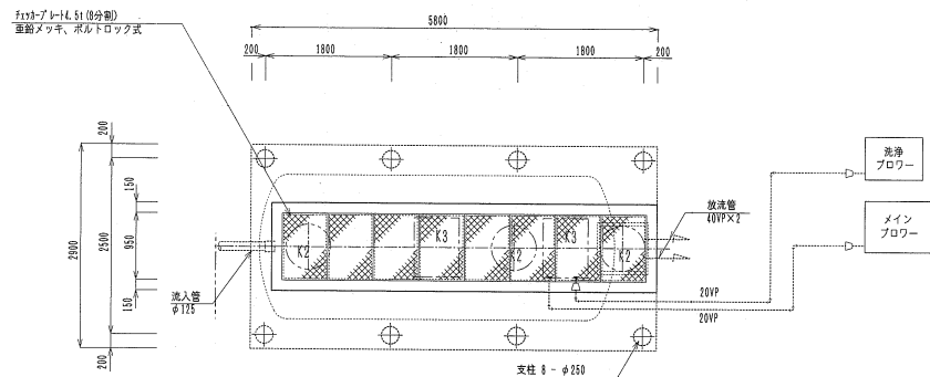
スラブ平面図
