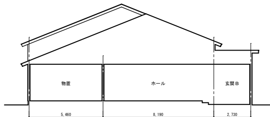
D-D 断面図 S=1/100
