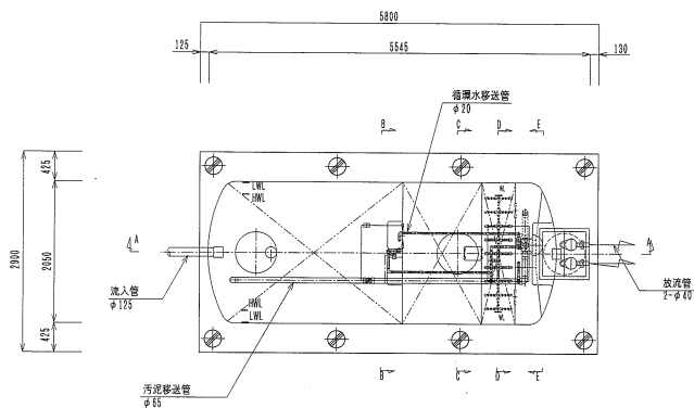
槽内部平面図
