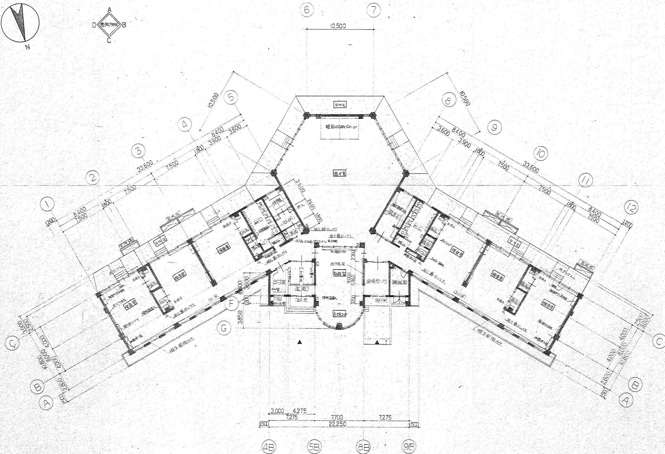
平面図 S-1.200 床面積 1209.78㎡
