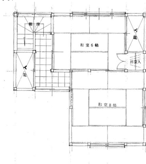
■ 間取2F
